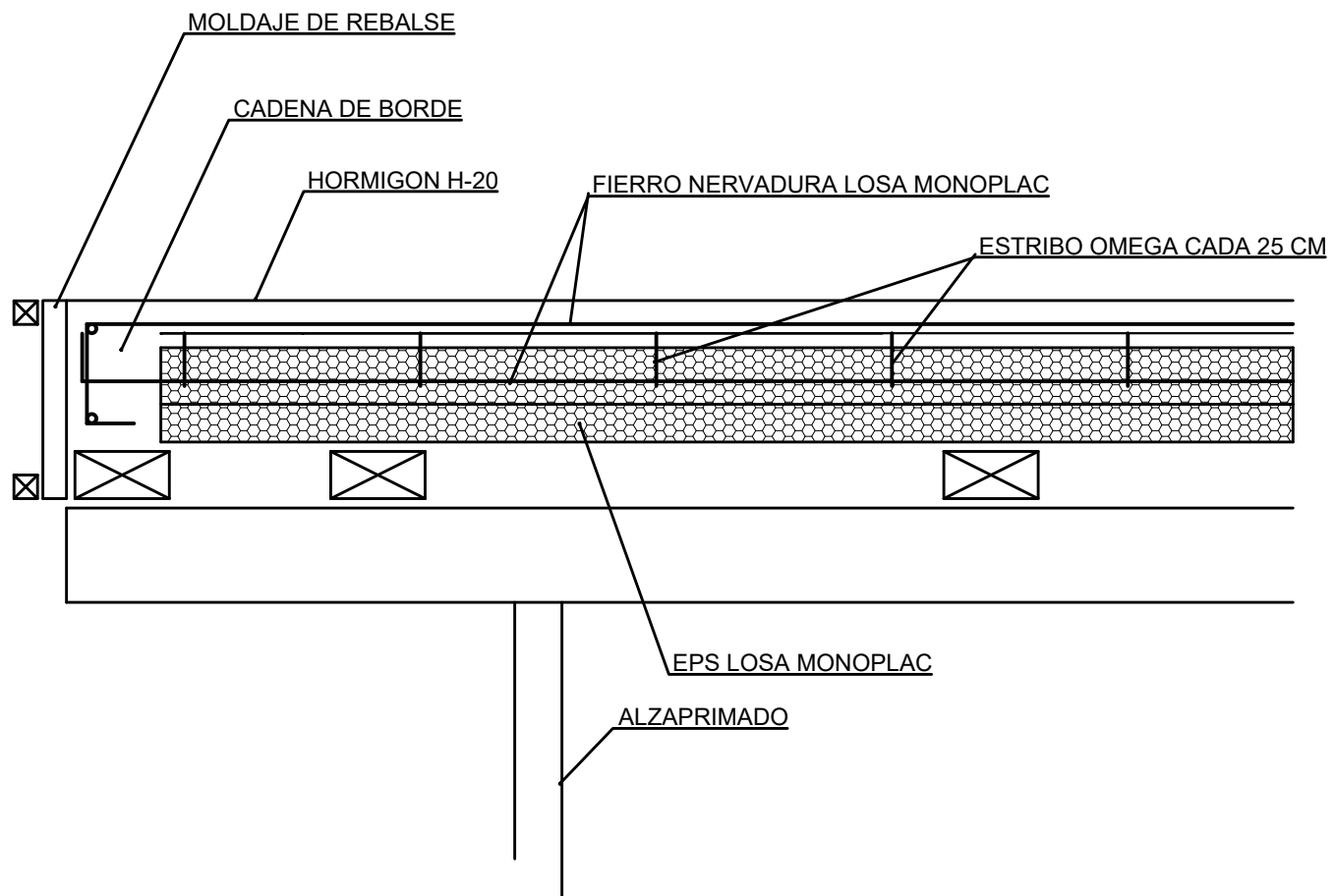
LOSA MONOPLAC EN VOLADO
