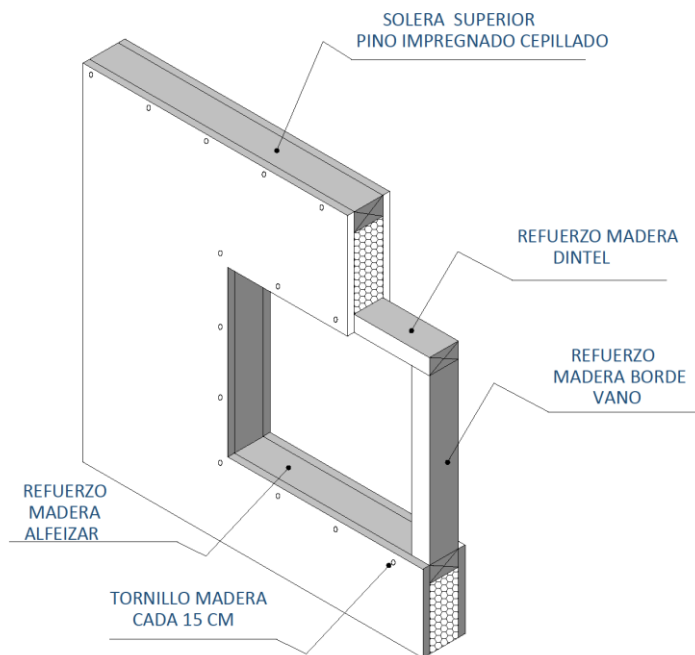
REFUERZO VANO
